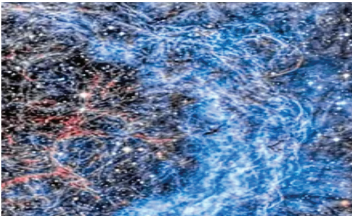
Filamentos gás brilhante
