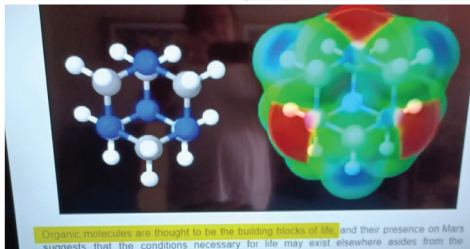
Telescópio James Webb identifica molécula orgânica em nuvem molecular
