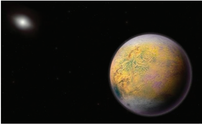
Recriação do planeta X.
